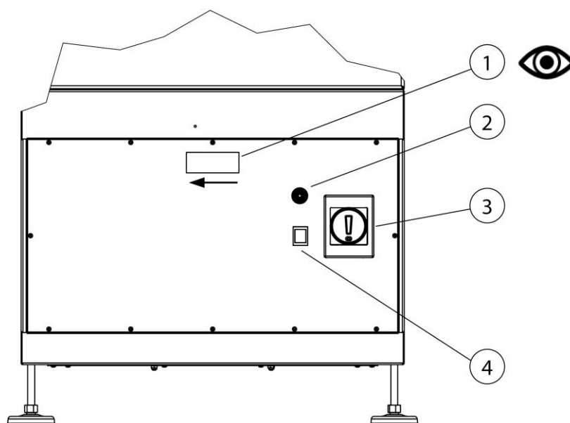
Fig. 5: Kontrollere rotasjonsretning på viften
