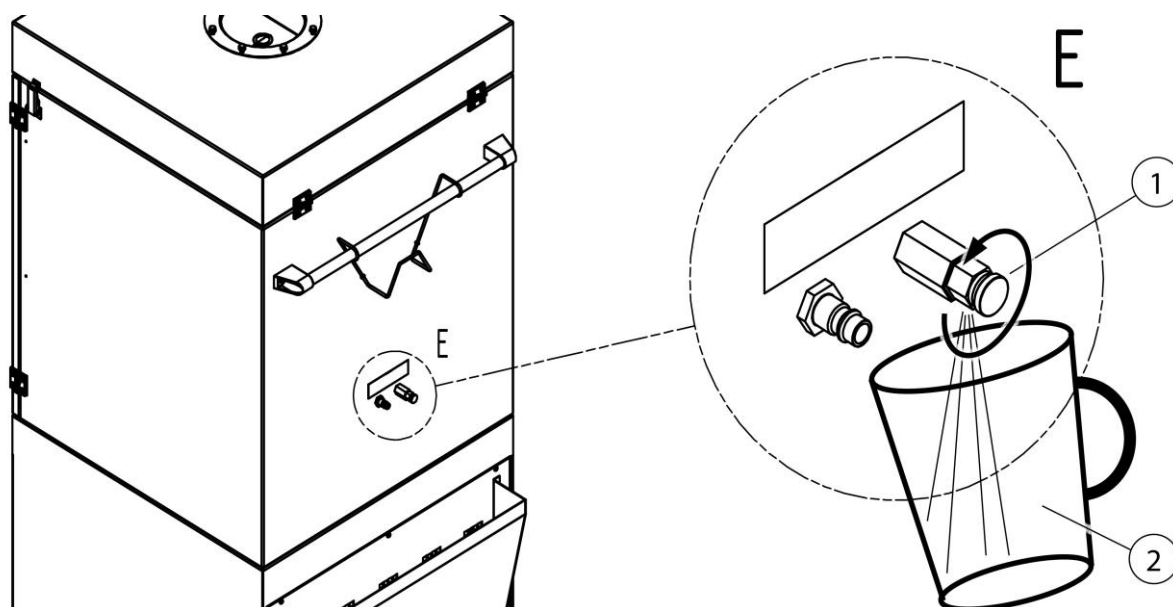
Fig. 8: tappe kondensat
