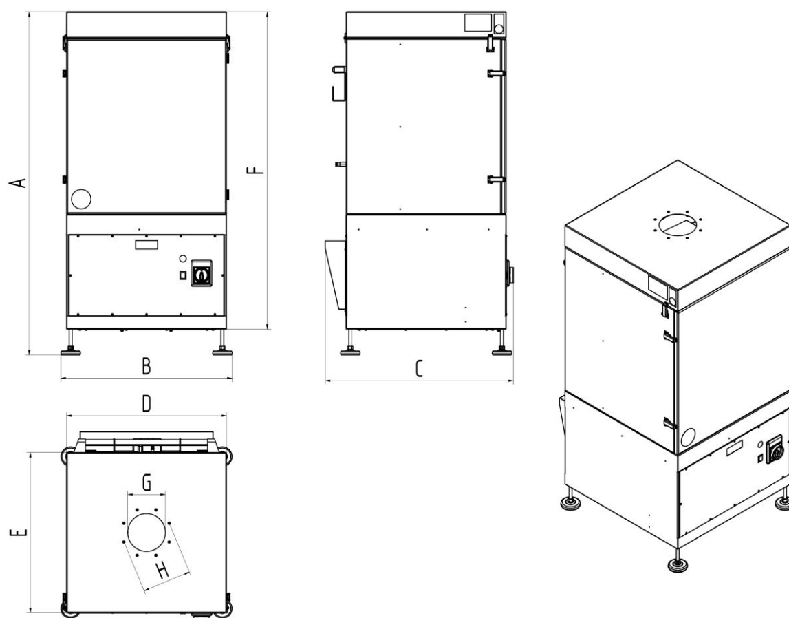
Fig. 13: Målskisse
