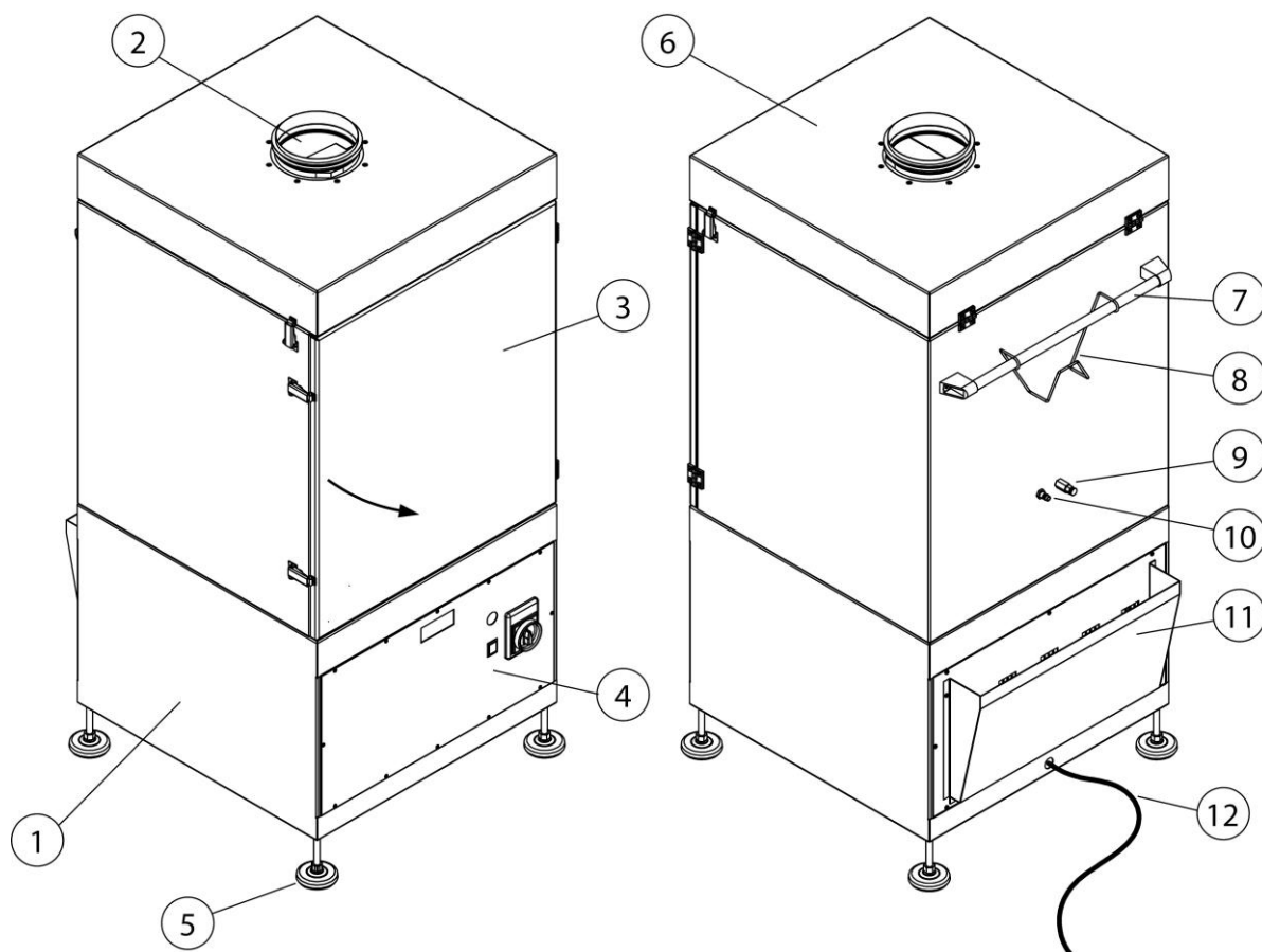
Fig. 1: Funksjonsbeskrivelse
