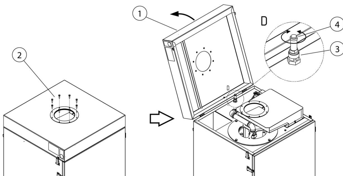
Fig. 12: Tilgang til sikkerhetsventil for trykkluft
